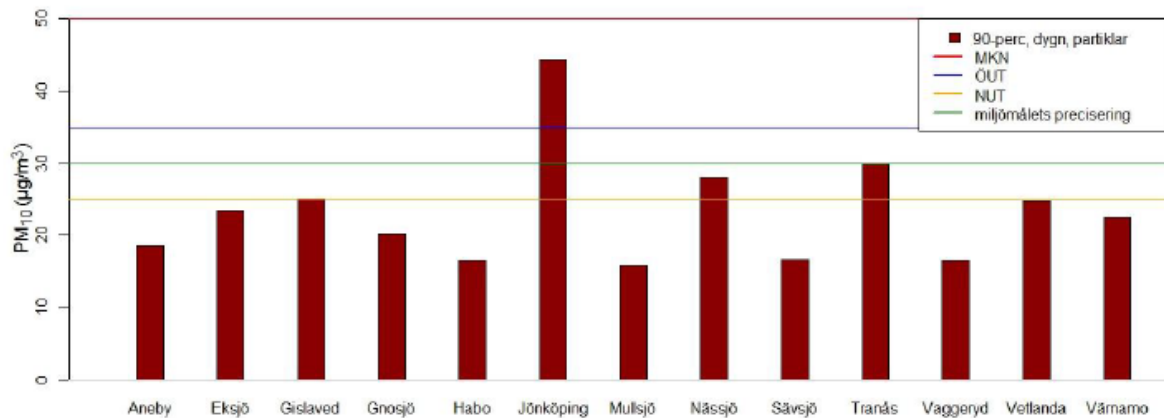
Figur 11 Högsta beräknade 90-percentil för dygnsmedelhalt av PM 10 i respektive kommun. Horisontella linjer indikerar miljö kvalitetsnormen (MKN), övre och nedre utvärderingströskeln (ÖUT och NUT) samt miljö kvalitetsmålets precisering för 90-percentil för dygnsmedelhalt.
